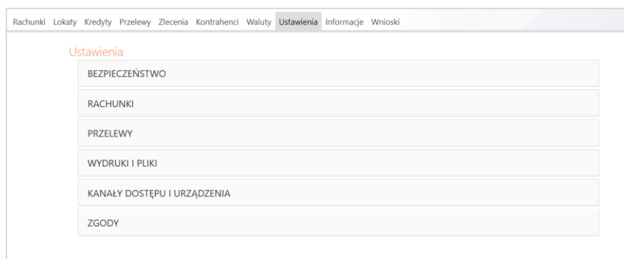
Rys. 43 Okno „Ustawienia”
